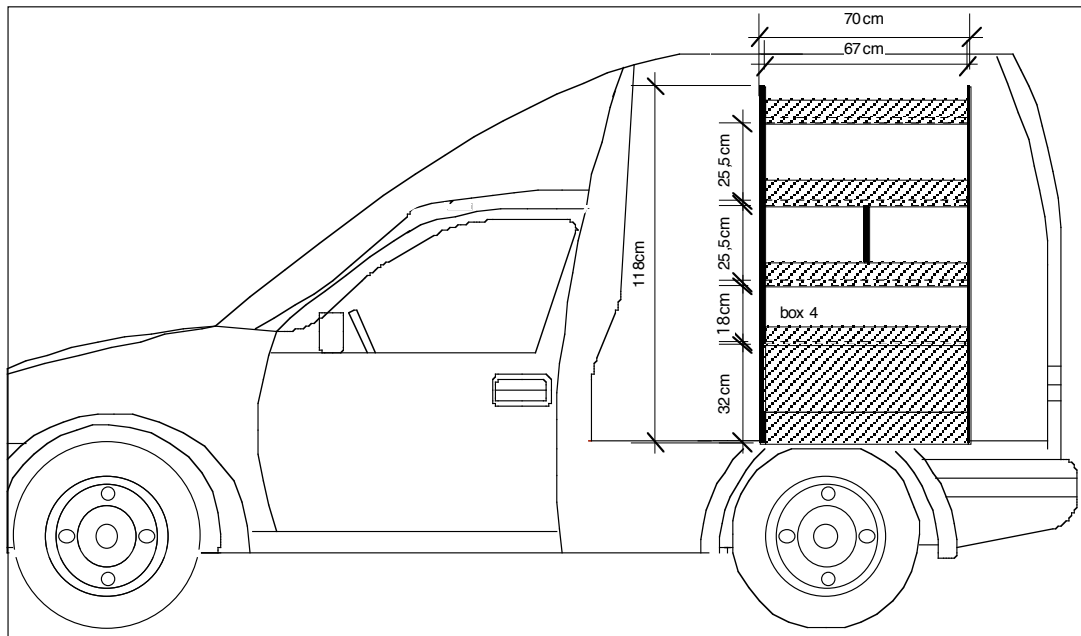
AGENCEMENT CADDY (TRADE ADVANCE) VUE DROITE
