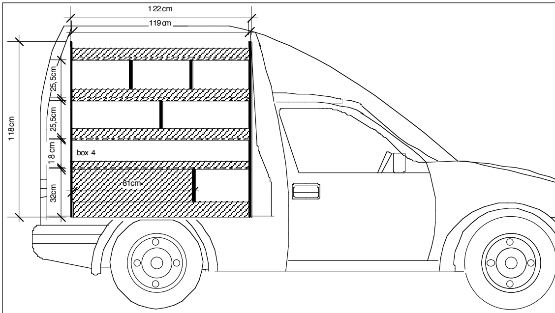
AGENCEMENT CADDY (TRADE ADVANCE) VUE GAUCHE
