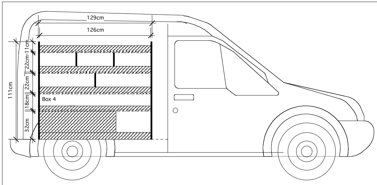
AGENCEMENT FORD CONNECT COURT (TRADE ADVANCE) VUE GAUCHE
