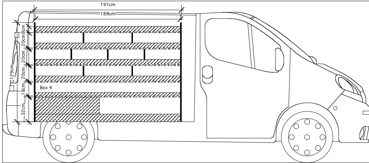
AGENCEMENT TRAFIC/VIVARO/PRIMASTAR L1H1 (TRADE ADVANCE) VUE GAUCHE
