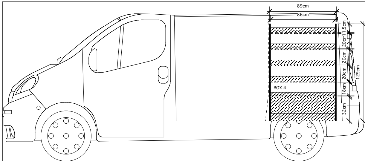
AGENCEMENT TRAFIC/VIVARO/PRIMASTAR L1H1 (TRADE ADVANCE) VUE DROITE
