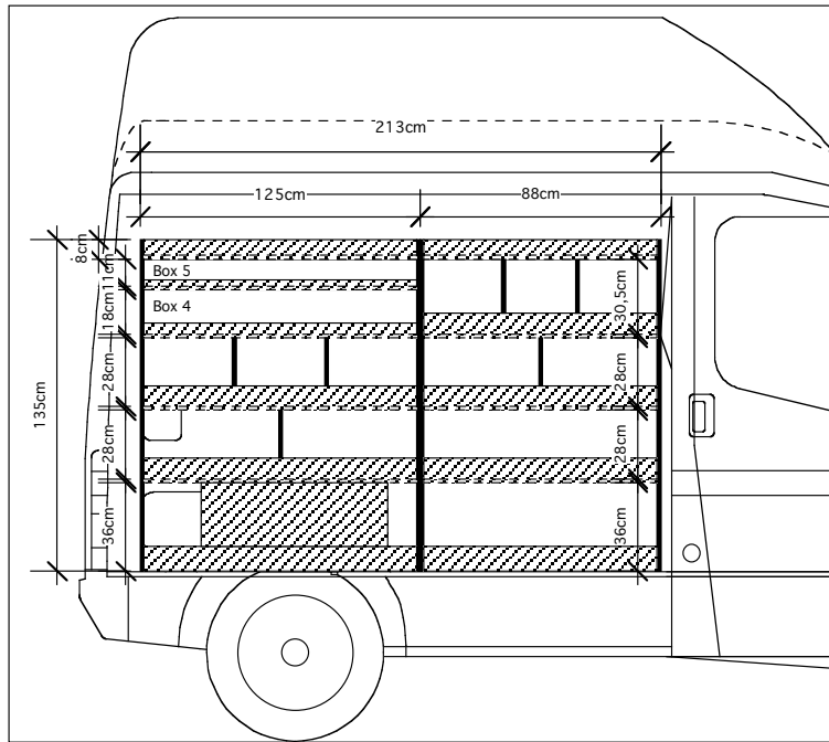
AGENCEMENT TRANSIT COURT BAS (TRADE ADVANCE) VUE GAUCHE
