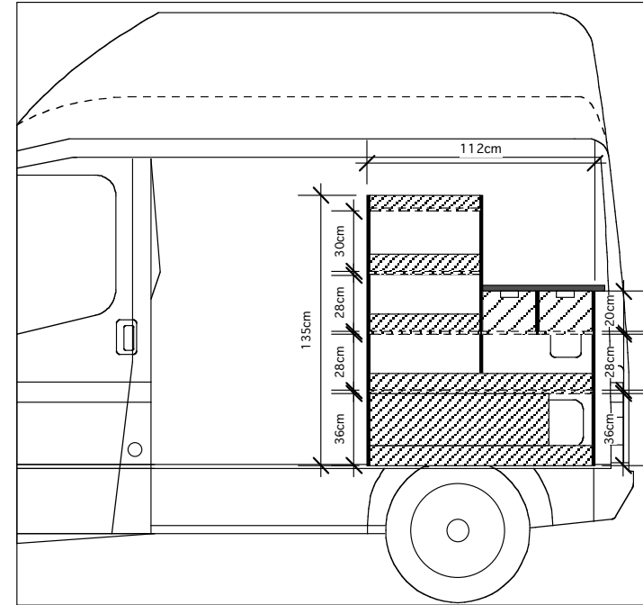
AGENCEMENT TRANSIT COURT BAS (TRADE ADVANCE) VUE DROITE
