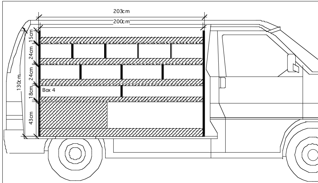
AGENCEMENT TRANSPORTER T5 COURT (TRADE ADVANCE) VUE GAUCHE
