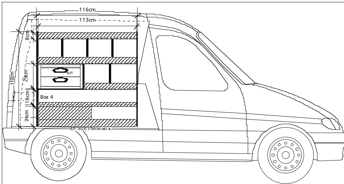
AGENCEMENT BERLINGO/PARTNER/KANGOO PL (TRADE ADVANCE) VUE GAUCHE
