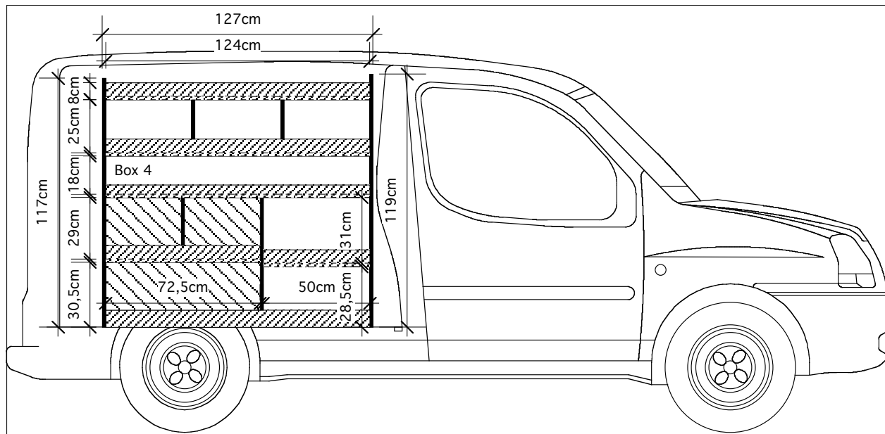
AGENCEMENT DOBLO COURT PL (TRADE ADVANCE) VUE GAUCHE
