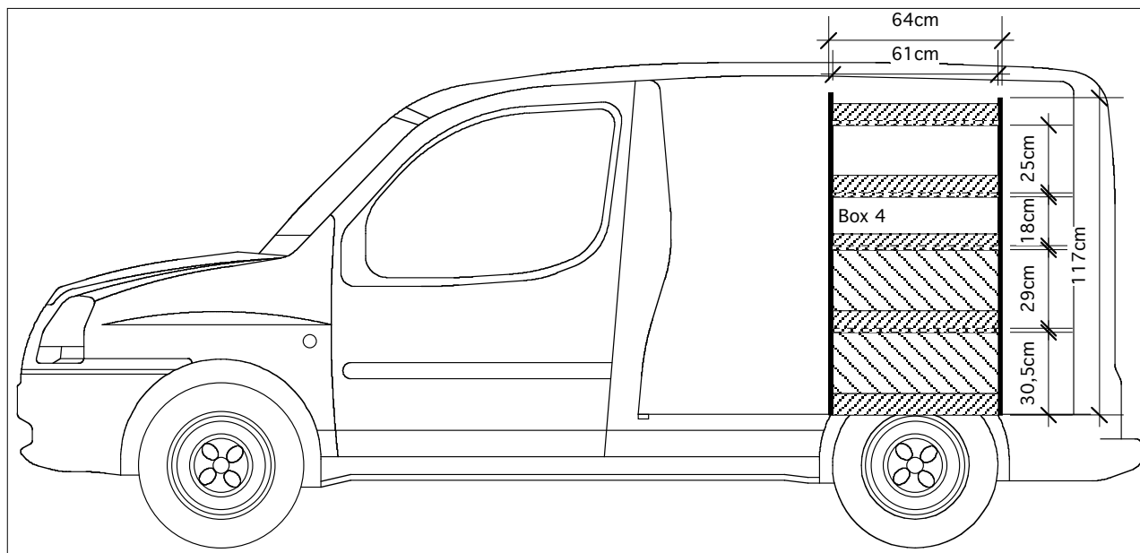
AGENCEMENT DOBLO COURT PL (TRADE ADVANCE) VUE DROITE
